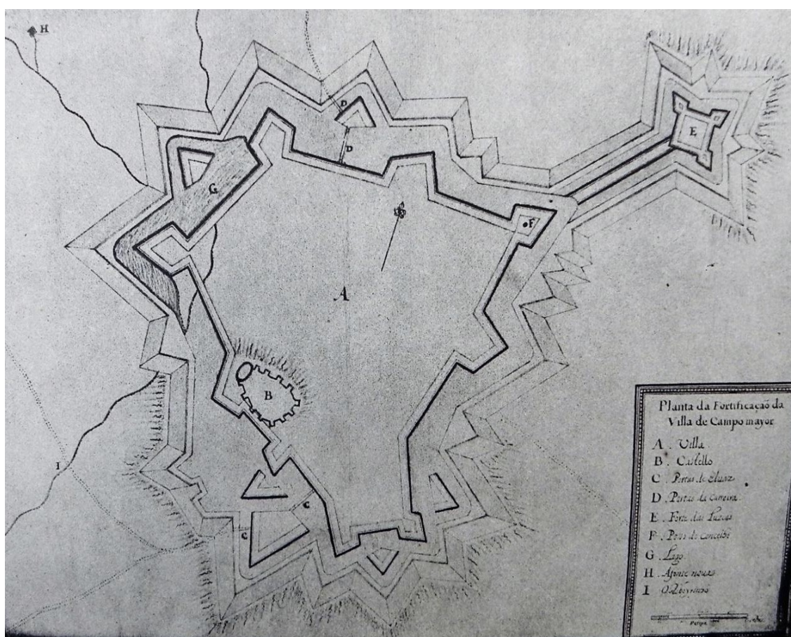
Fig. 14. Plano de Campo Maior ( Livro das Praças de Portugal com suas fortificações. Desenhadas pelos Engenheiros de Sua Magestade Cosmander, Gilot, Langres, Santa Colomba & outros delineadas por João Nunes Tinoco, architecto de Sua Magestade, ano 1663, João Nunes Tinoco, apud MATOS, Gastão de Melo de, Nicolau de Langres em Portugal, Publicação da Comissão de História Militar, Lisboa, 1941, lám. LXXXI ).
